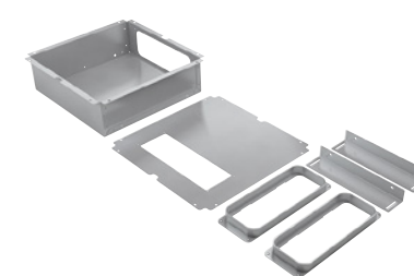
LZ29IDP00 Standard kulfiltersæt – Long Life Startsæt til brug for recirkulation. Standard kulfilter. Levetid: 12 måneder. Lugtreduktion: > 80 %. Regenereringsproces: 2 timer ved 200 °C i ovnen hver 4. måned. Indeholder 2 kulfiltre, fleksslange og 2 monteringsrammer. Vejl. pris kr. 2 072
